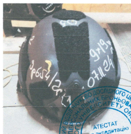
Фото 2 (зразок 654/2 після випробувань)
